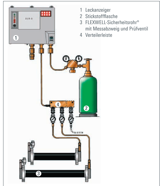
Überdruckleckanzeigesystem
